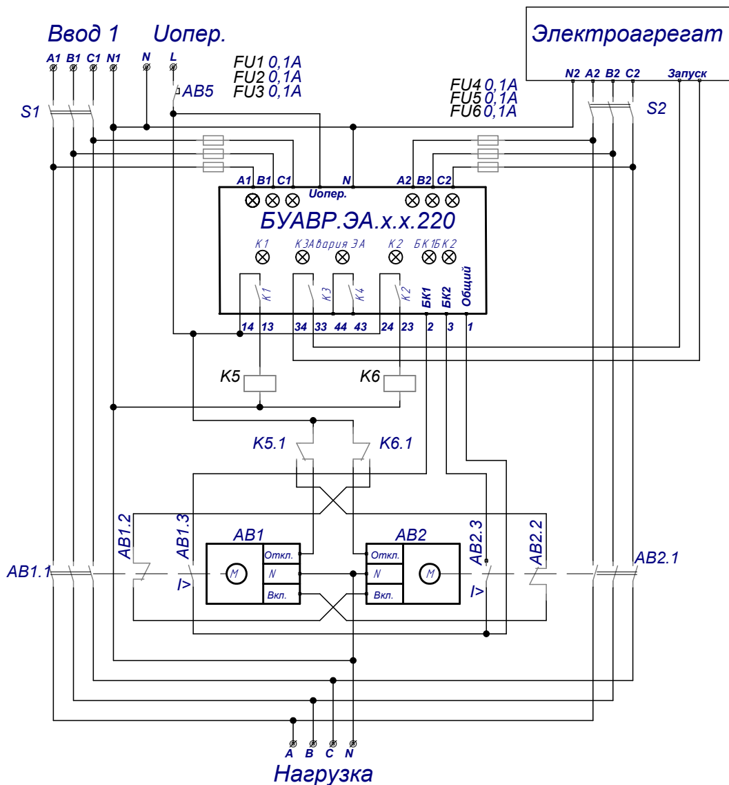
Рис.6 Схема АВР на автоматических выключателях с мотор-приводом, двумя вводами, один из которых электроагрегат, одной нагрузкой, электрической блокировкой автоматических выключателей, блокировкой по цепям максимальной токовой защиты автоматических выключателей и управлением от БУАВР.ЭА
